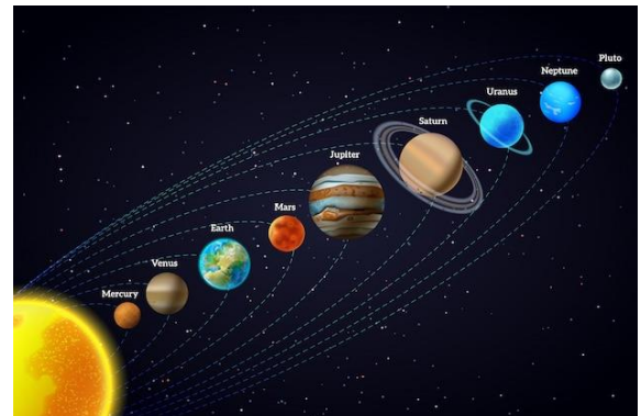
Sonnensystem Bild: macrovector Quelle: freepik.com
